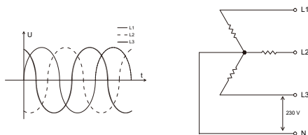
Abbildung 230 / 400V dreiphasiges WYE-Stromnetz und Anschluss jedes Ports
