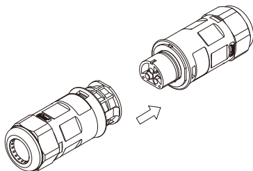
Abbildung Schließen Sie den Netzstecker an
