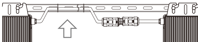
Abbildung Befestigen Sie die AC-Kabel
