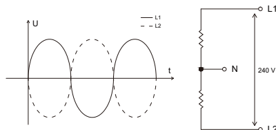
Abbildung Zweiphasiges Split-Stromnetz und Anschluss jedes Ports
