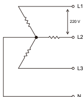
Abbildung 127 / 220V dreiphasiges WYE-Stromnetz und Anschluss jedes Ports
